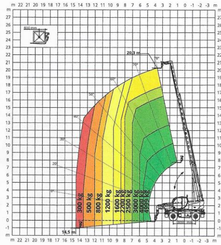
JIB 2.000 kg
