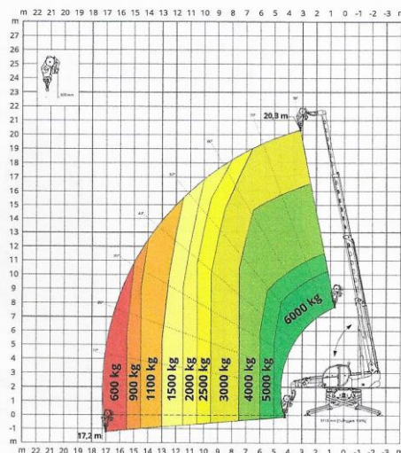
GANCIO 6.000 kg
