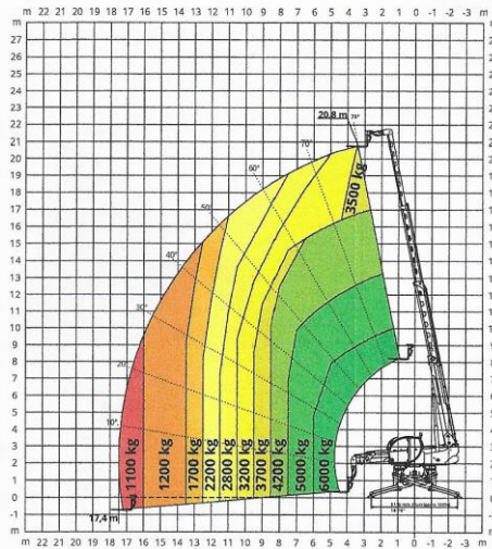
ARGANO 6.000 kg
