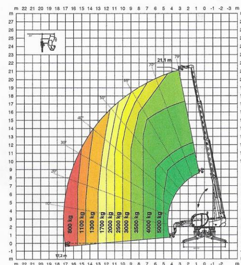
GANCIO 6.000 kg
